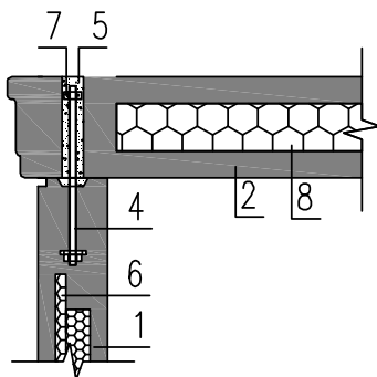
(c) 墙板与楼板顶层处连接
