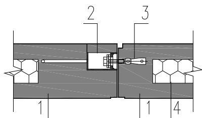
图6.5.7-1 楼板与楼板连接
