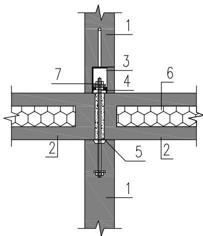
(a) 预制隔墙板与楼板连接
