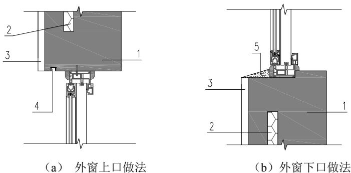
图 5.3.6 窗洞口构造示意
