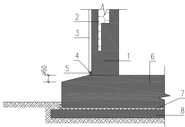
图 5.2.2 基础、地面和首层外墙防水（防潮）构造示意
