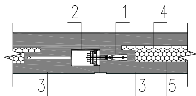
(a) 预制墙板与墙板一字连接
