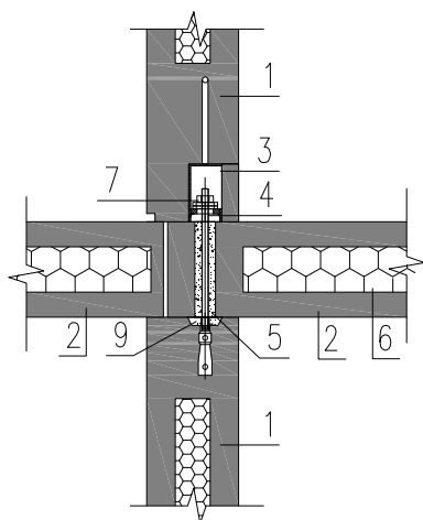
(b) 预制墙板与楼板连接
