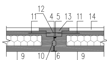
(f) 屋面板拼缝
