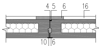
(c) 外墙水平缝
