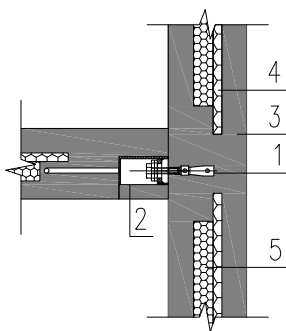
(c) 预制墙板与墙板 T 连接
