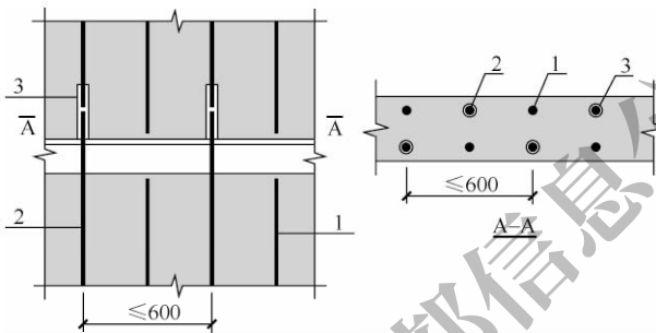
图 5.7.10-1 竖向分布钢筋“梅花形”套筒灌浆连接构造示意 1—未连接的竖向分布钢筋；2—连接的竖向分布钢筋；3—灌浆套筒
