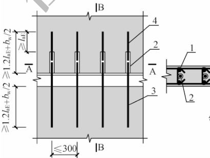
图 5.7.10-2 竖向分布钢筋单 1—上层预制剪力墙竖向分布钢筋；2— 4—上层剪力墙连接
