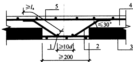
图 6.6.6 双向叠合板整体式接缝构造示意
