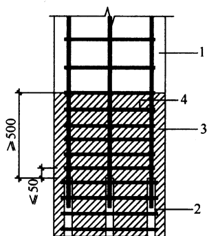
图 7.3.5 钢筋采用套筒灌浆连接时柱底箍筋加密区域构造示意
